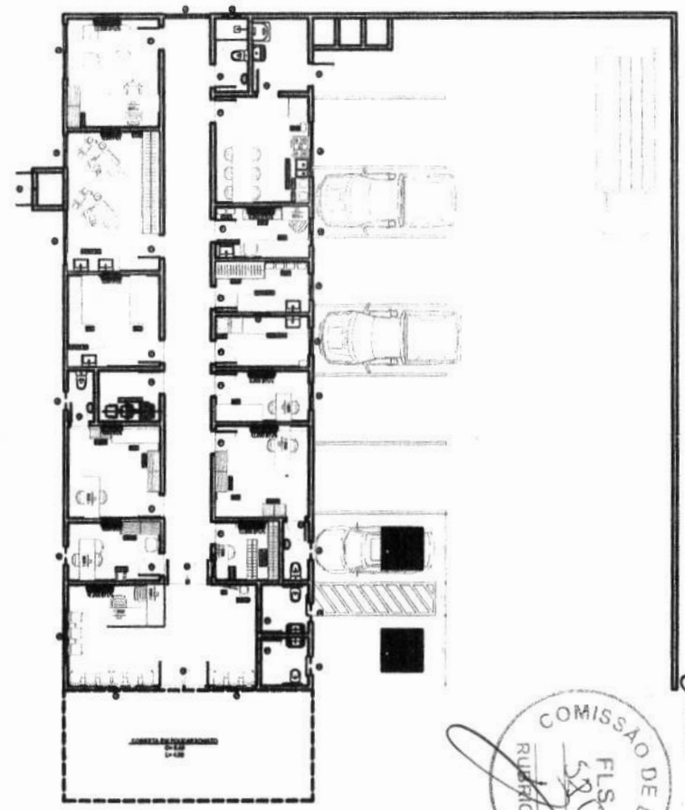
LAYOUT ESCALA: 1/150
